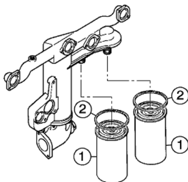
Рис. 9. Масляный фильтр:
