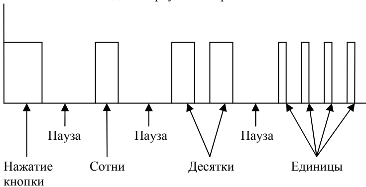
Рис. 31. Пример блинк-кода 1-2-4 (пониженное напряжение бортовой сети)
