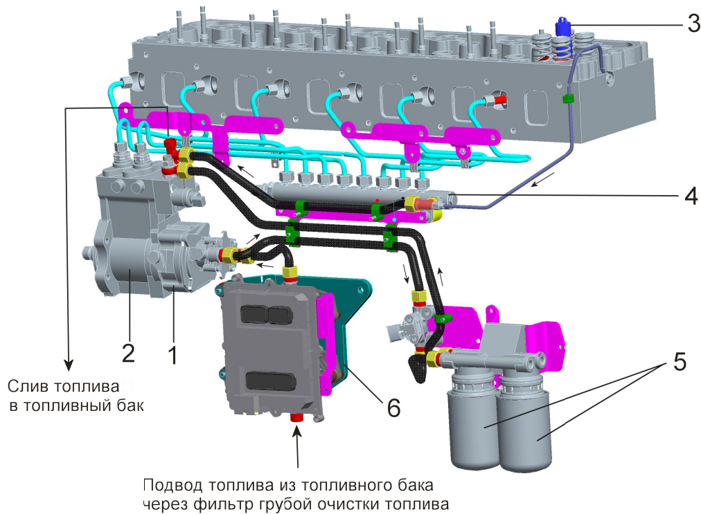
Рис. 8. Топливная система «Common Rail»:
